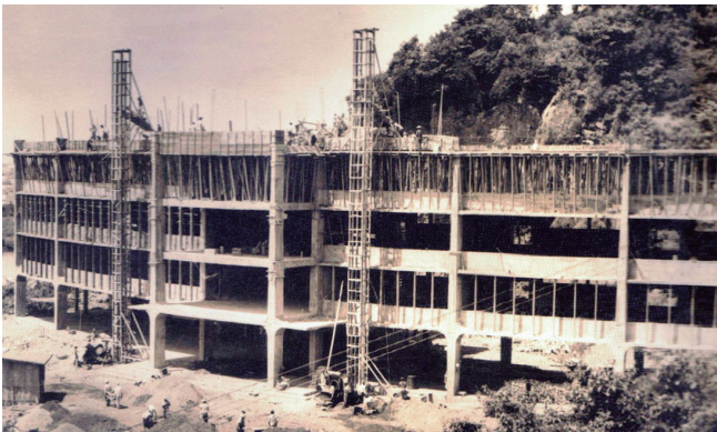
Figura 4 Construcción del edificio principal de la UCSG Biblioteca General “Dr. Francisco Illescas Barreiro” UCSG
